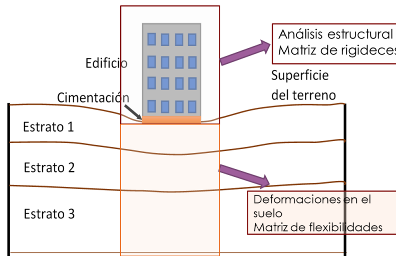
Figura 1.1. Compatibilidad de deformaciones
