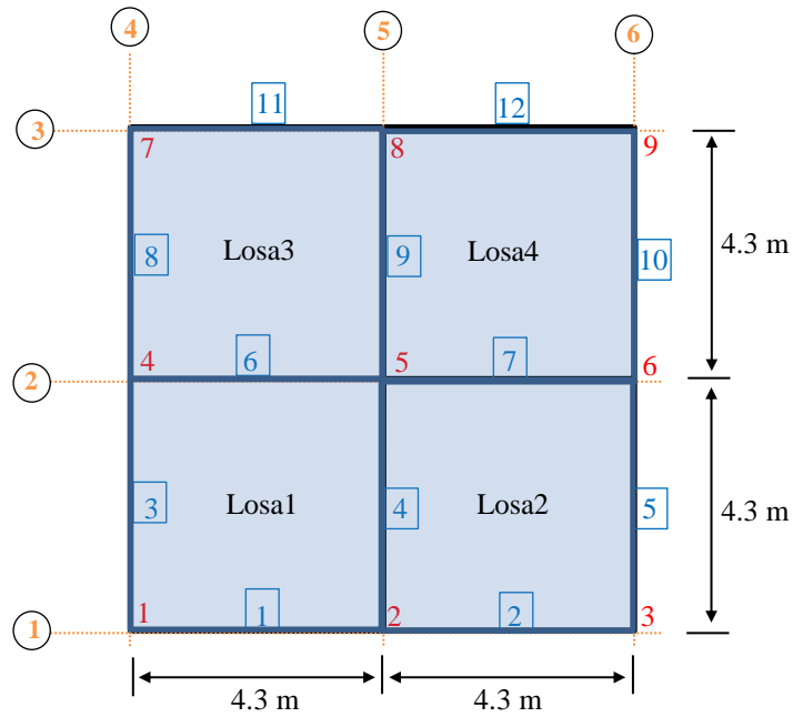
Figura 7.3.2. Idealización de la subestructura
