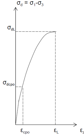
Figura 4.1 Curva esfuerzo-deformación unitaria no lineal
