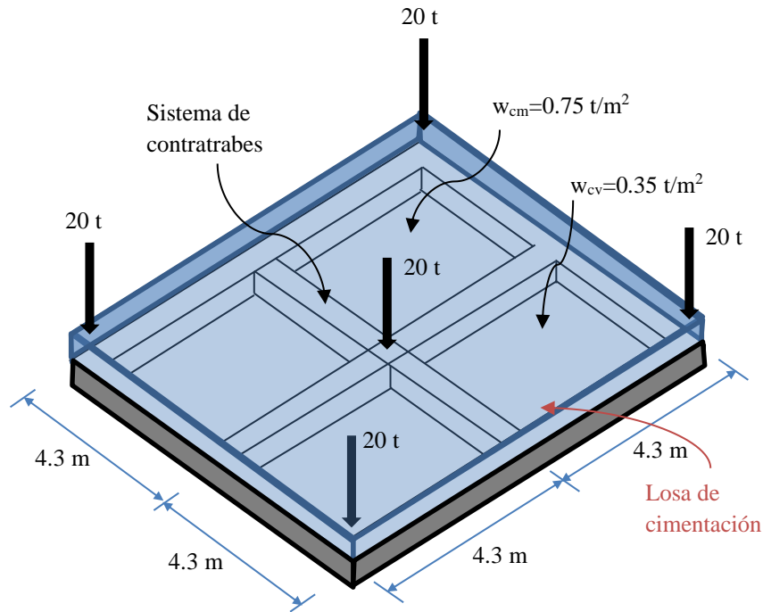
Figura 7.3.1. Sistema de cimentación basada en losa sobre zapatas corridas
