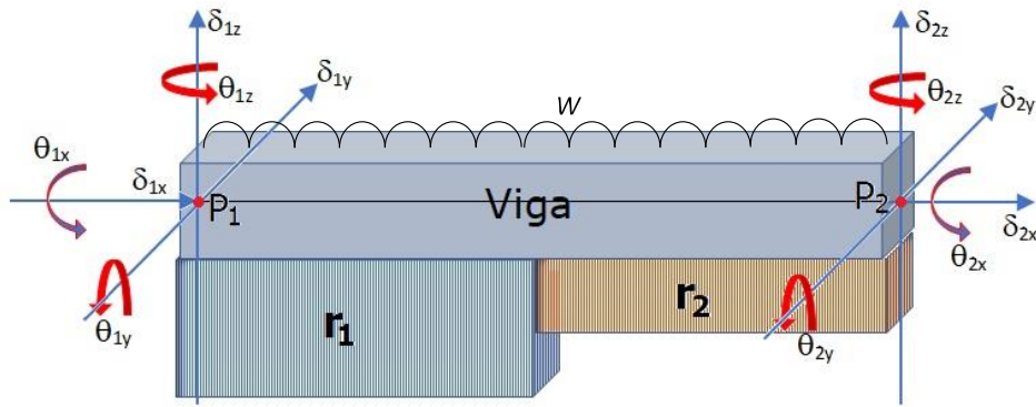
Figura 2.2. Desplazamientos, cargas y reacciones del suelo considerados en una barra de cimentación. r_1 y r_2 son las reacciones hipotéticas del suelo actuando sobre la barra de cimentación.
