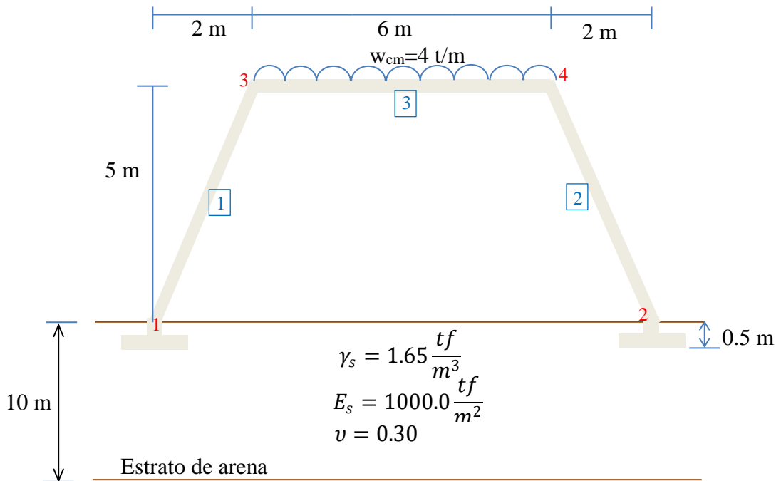
Figura 7.1.1 Marco bidimensional, inclinado y con zapatas aisladas
