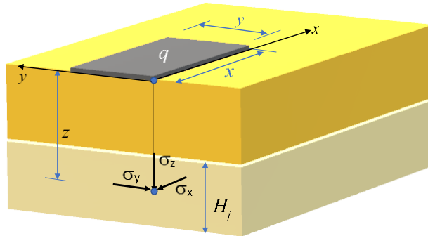
Figura 3.1. Incrementos de esfuerzos normales bajo la esquina de un rectángulo cargado uniformemente en un medio semi-infinito.
