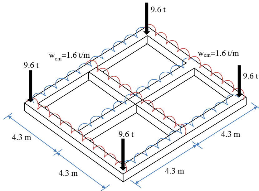
Figura 7.2.1. Sistema de cimentación basada en zapatas corridas
