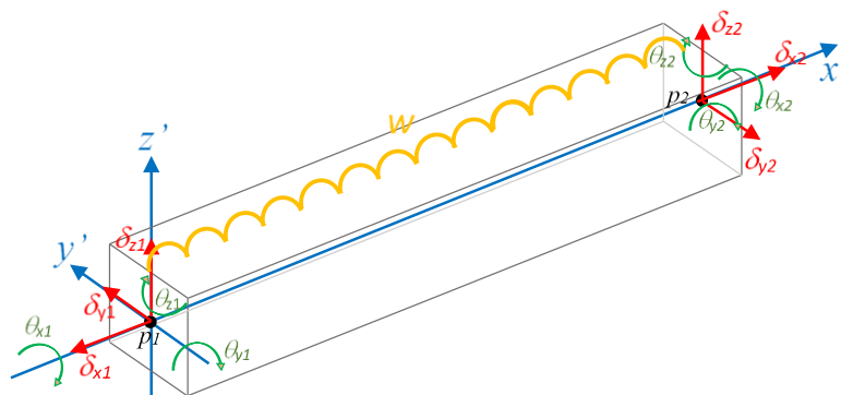
Figura 2.1. Cargas y desplazamientos considerados en una barra
