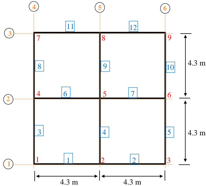
Figura 7.2.2. Idealización de la subestructura
