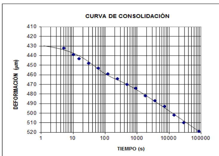
Figura 1. Curva de consolidación
