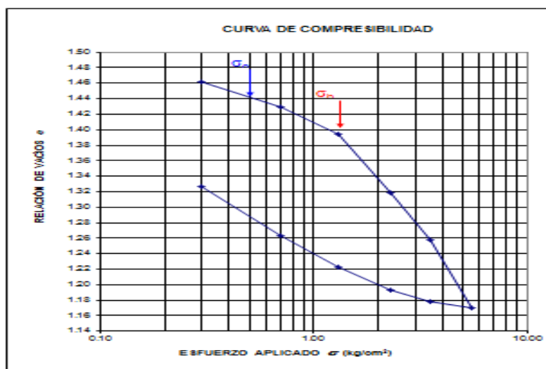
Figura 2. Curva de compresibilidad.
