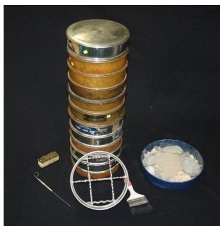
Figura 2. Equipo empleado.
